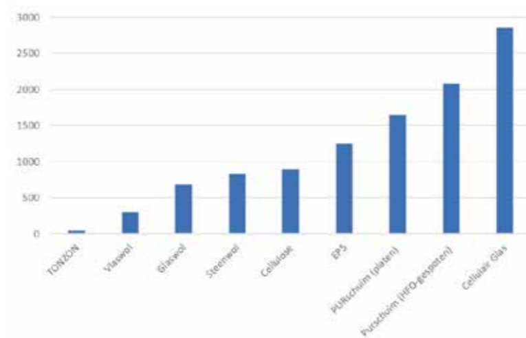
Uitstoot kg CO2 eq. bij 46m 2 vloerisolatie met Rc=7 m 2 K/λ
